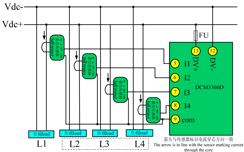
直流正系统接法 DC positive system connection
