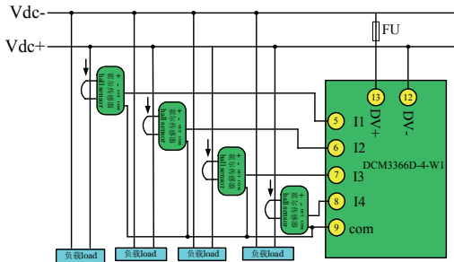
直流正系统接法 DC positive system connection
