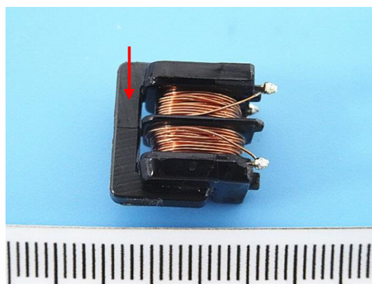
4.34 (客户参考图片 (非测试样品)) (Client Reference Photo(Non-tested sample))
