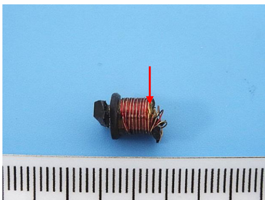
2.32 (客户参考图片 (非测试样品)) (Client Reference Photo(Non-tested sample))
