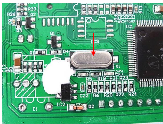
3.13 (客户参考图片 (非测试样品)) (Client Reference Photo(Non-tested sample))
