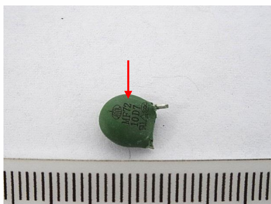
4.49 (客户参考图片 (非测试样品)) (Client Reference Photo(Non-tested sample))
