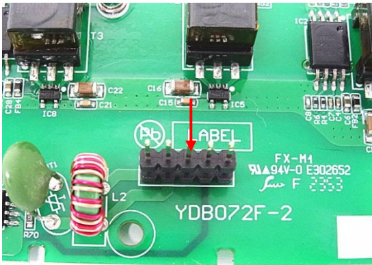
2.8 (客户参考图片 (非测试样品)) (Client Reference Photo(Non-tested sample))
