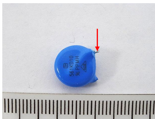
4.54 (客户参考图片 (非测试样品)) (Client Reference Photo(Non-tested sample))
