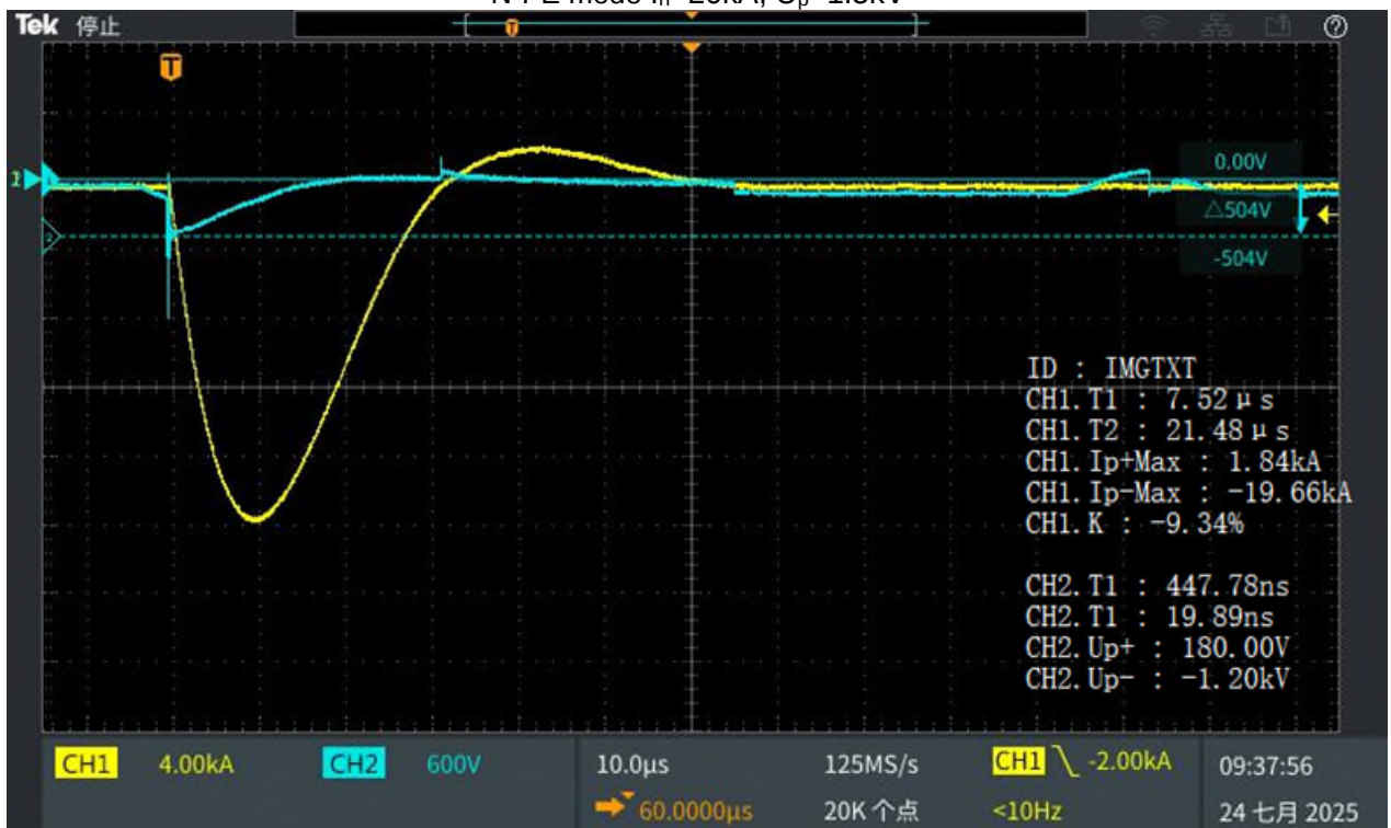
N-PE mode I_n=20\text{kA} , U_p=1.5\text{kV}
